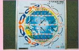
3421 大氣環流演示模型 62x66cm
