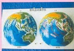
3426 季風活動演示模型 44x83cm
